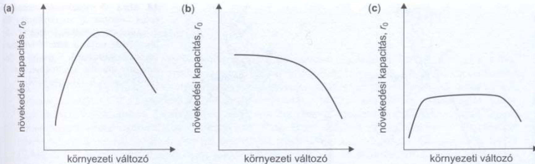
13. ábra Válaszgörbe-típusok.
