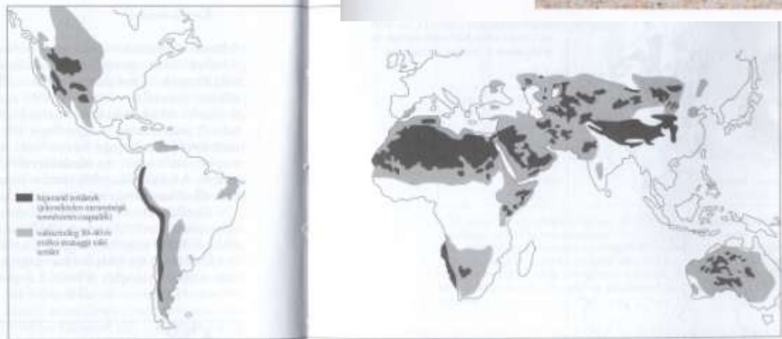
7.7. ábra. A Föld arid régióiban egyre nagyobb területeket hódít el a sivatag (Allan & Warren 1993) A feketével jelölt területek már bioparadisek, minimális csapadékkal. A szürke színezés az elővártékező évtizedekben az elsivatagosodás veszélyének kitétt területeket jelöli.
