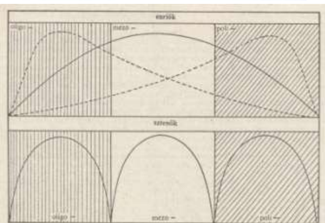
107. ábra: Az élőlények csoportosítása töréshatárak szerint (Wurmbech nyomán)
