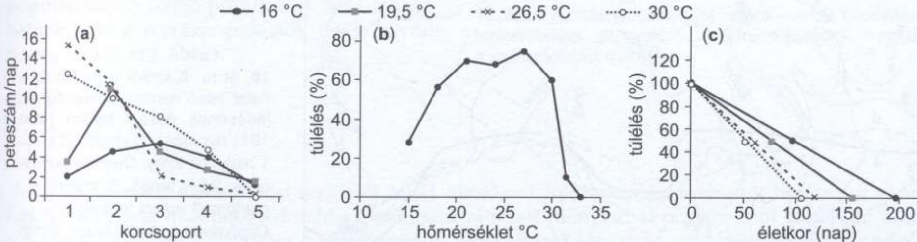
9. ábra Az amerikai kukoricabogár hőmérsékletfüggő életmenet-komponensei. (a) Peteszám korcsoportgörbék hőmérsékletfüggése, (b) túélés hőmérsékletfüggése, (c) élethossz hőmérsékletfüggése (HEMERIK és mtsai 2004 nyomán).
