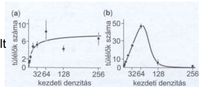
29. ábra Pontosán kompenzált (a) és túlkompenzált (b) denzitásfüggés bogaraknál. A pontok az átlagot, a bajuszok a szórást jelölik. (a) Stegobium paniceum , (b) Lasioderma serricorne (BELLAWS 1981).
