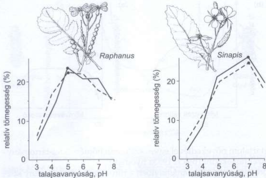
14. ábra A mézskerülő repcsény retek ( Raphanus raphanistrum ) és a vadrepce ( Sinapis arvensis ) válaszgörbéi egyfajú veteményekben (monokulturában). Egy-egy vonal egy-egy kísérlet eredménye (MULLER-DOMBOIS, ELLENBERG 1974).
