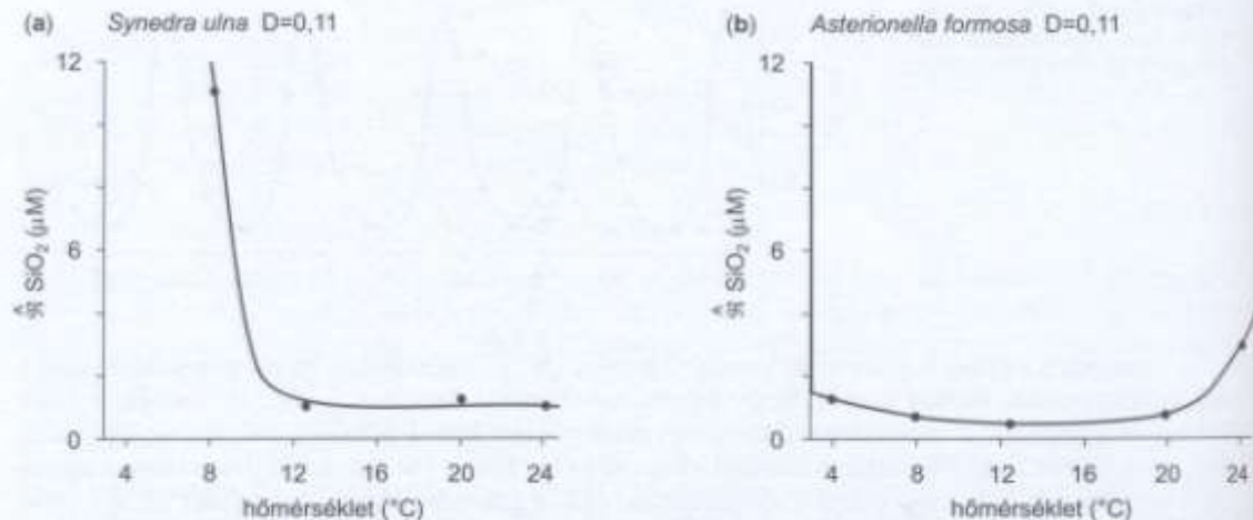
18. ábra A S. ulna (a) és A. formosa (b) kovamoszat-tenyészetek egyensúlyi szilícium-dioxid-koncentrációja ( \mu\text{SiO}_2 (μM)) különböző hőmérsékleteken. Egy-egy pont két monokultúrában mért koncentráció átlaga (TILMAN és mtsai 1981).
