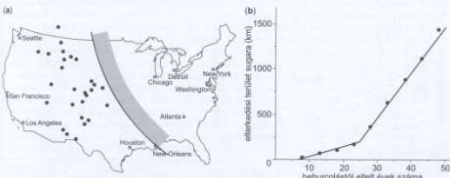
21. ábra Európai seregek elterjedése (a) terjedési front és szóróvonal előfordulások (•), (b) elterjedési terület változása az idővel.
