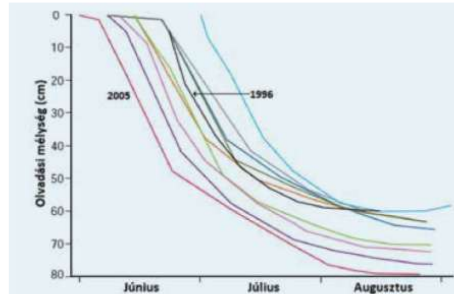
25TA7/3. ábra. A permafroszt felolvadási mélysége a nyári hónapokban Grönlandon egy 10 éves periódusban. Minden görbe 121 mérési pontból készült. A legkorábbi év 1996 (fekete), az utolsó 2005 (piros), a közbűlő évek más-más színűek [Christiansen és mtsai (2008) nyomán módosítva].
