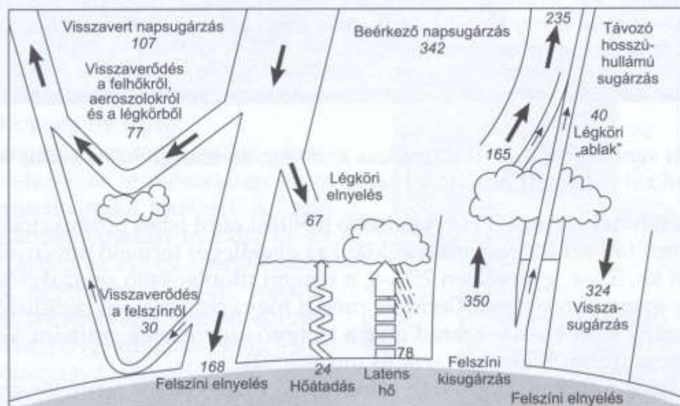
4. ábra A Föld energiámérlege. A légkör külső határára érkező napsugárzás egy része (31%, 107 \text{ W/m}^2 ) közvetlenül, rövidhullámú sugárzás formájában verődik vissza (a légkörben található, számottevő felszínnel rendelkező részecskékről, a felhőzetről vagy a Földfelszínről), nagyobbik hányada viszont (69%, 235 \text{ W/m}^2 ) bolygónk felszínéről hosszúhullámú sugárzás formájában visszaverődve hagyja el a légkört. A légköri üvegházgázok elnyelik a felszínről visszaverődő infravörös sugárzást (az elektromágneses spektrum egy szűk tartománya, az ún. légköri „ablak” kivételével), majd minden irányban — beleértve a Föld felszínét is — visszasugározzák azt (üvegházhatás). A számértékek az energia mennyiségét mutatják \text{W/m}^2 egységekben (forrás: IPCC 2001).
