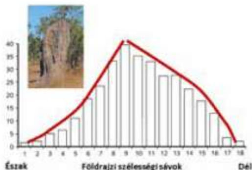
26/8. ábra. A termeszt (Isoptera) genusok száma földrajzi szélességi sávok mentén. Az adatok 611 ezer km 2 területű kvadrátokból származnak. Az Egyenlítő a 9. és 10. egység között helyezkedik el [Eggleton (1994) nyomán módosítva]. Fotó: Török János
