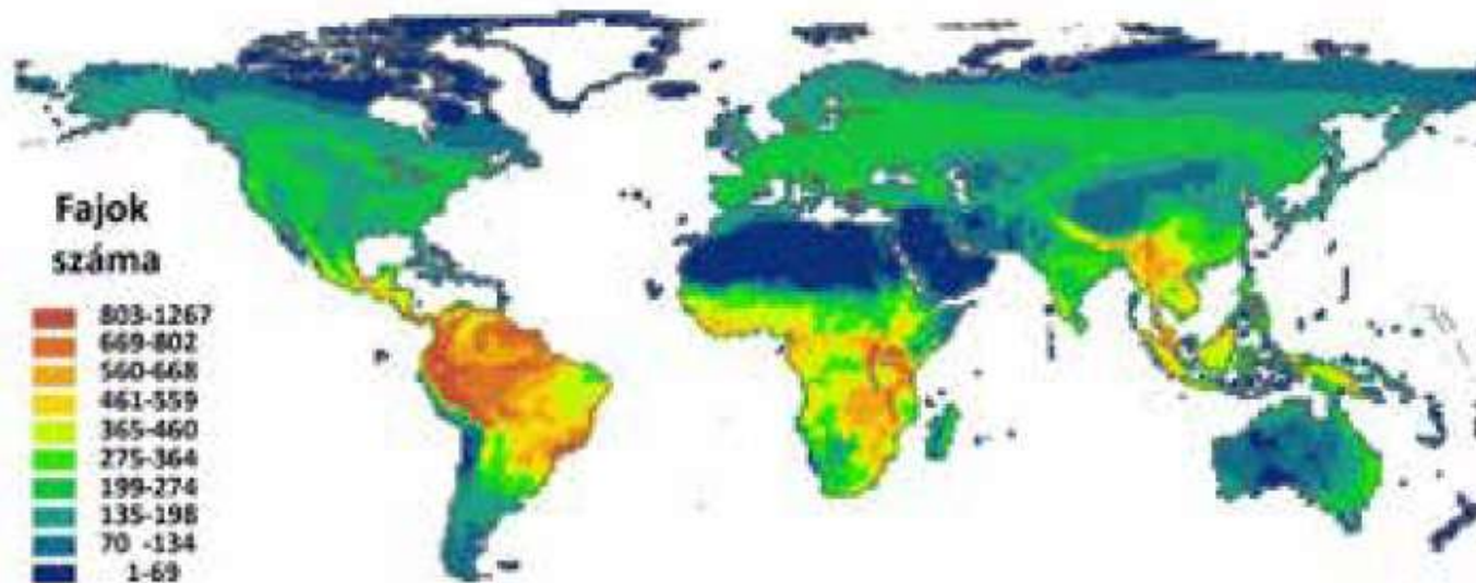
26/6. ábra. A szárazföldi kételtűek, madarak és emlősök együttes fajgazdagsága (fajok száma) a sarkoktól az Egyenlítő felé növekszik [www.biomac.org és Rahbek és mtsai (2019) nyomán módosítva].
